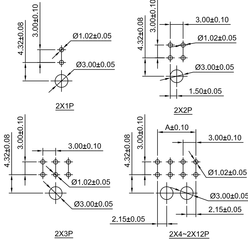
P.C.B LAYOUT
