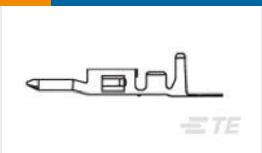
TE Part #794955-4 VAL-U-LOK PIN PHBZ AU 22-18AWG
