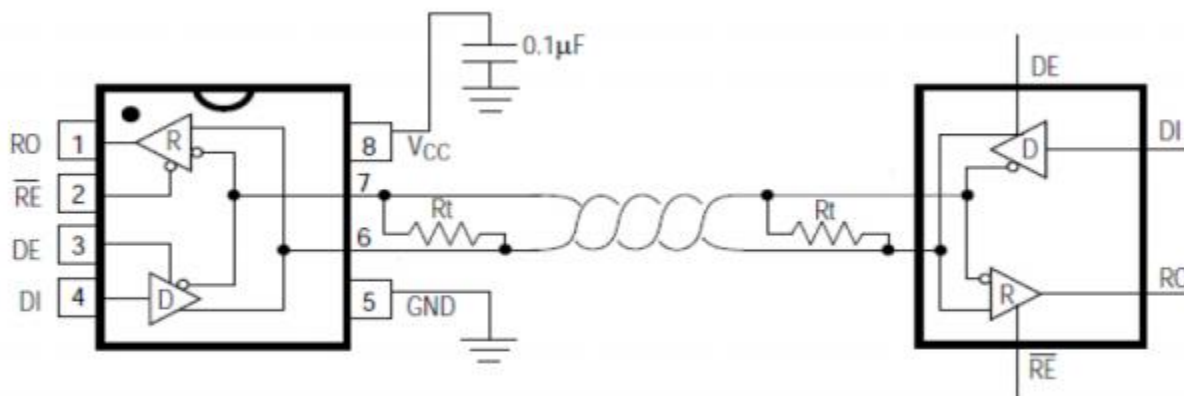
图 1：MAX485ESA典型半双工应用电路
