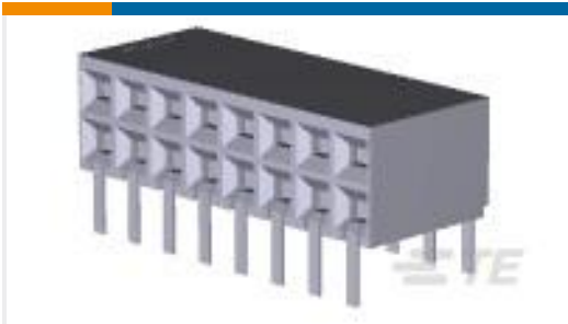
TE Part # 1-5535512-8 16 MODII HORZ DR CE EESS .100
