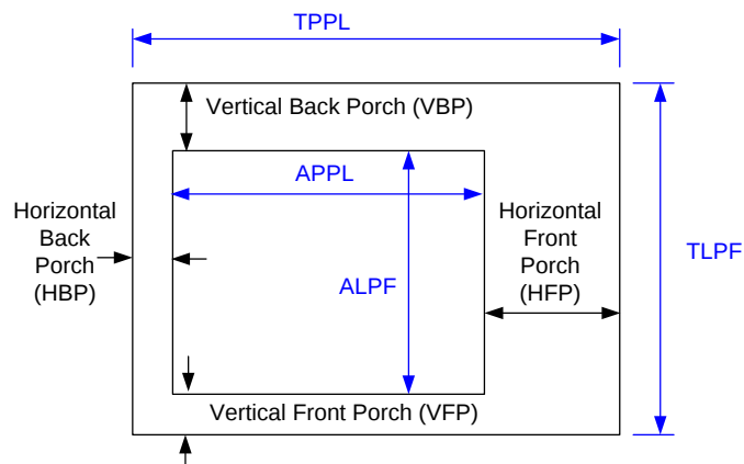
Figure 29. Timing Parameter Diagram
