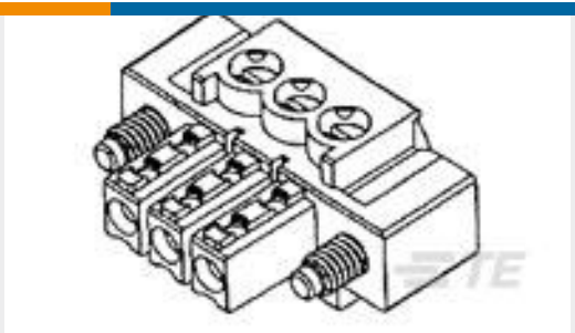
TE Part #1-284510-0 10P TERMI-BLOK PLUG CON VITI
