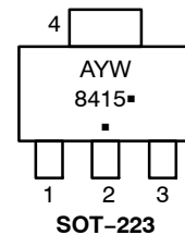
SOT-223
