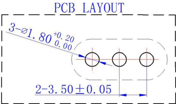
PCB 安装孔示意图
