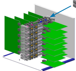
Cabled-Midplane
