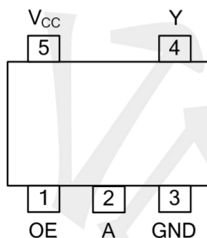
SOT353
