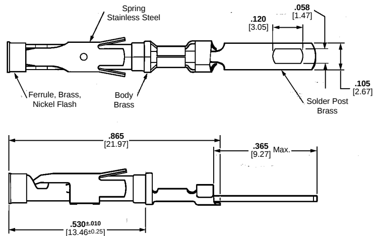
Socket
