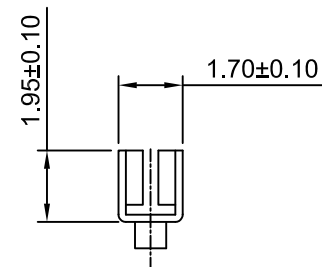
SEC:B-B
