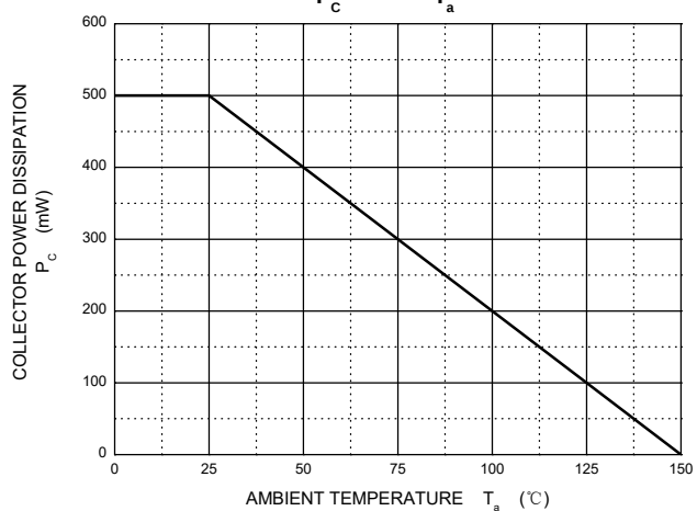
P_C — T_a
