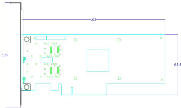
产品结构图
