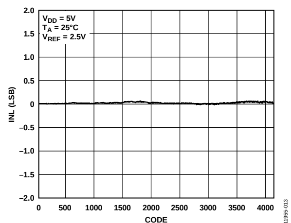
Figure 13. AD5681R INL
