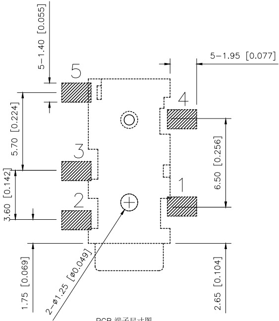
PCB端子尺寸图 TOP VIEW
