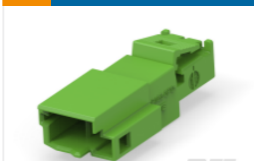
TE Part #2203701-3 2POS, MCON 1.2 CB TAB 2p TL UNSEALED
