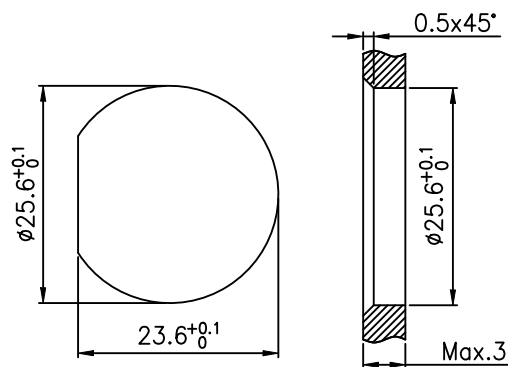
面板开孔尺寸
