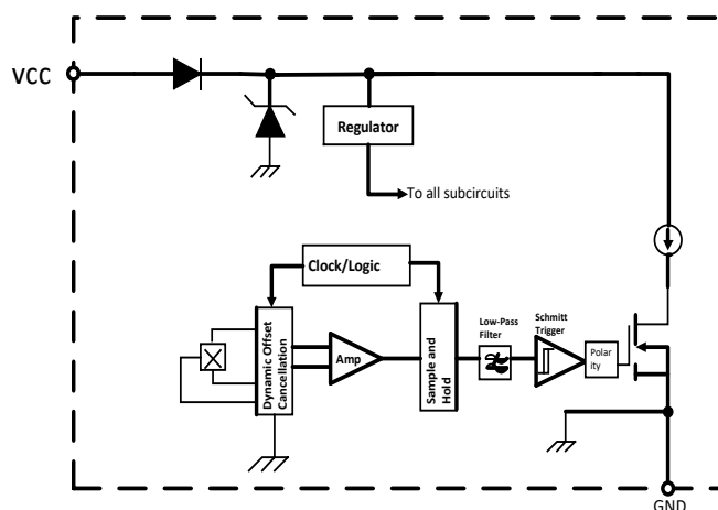
AH544 功能框图
