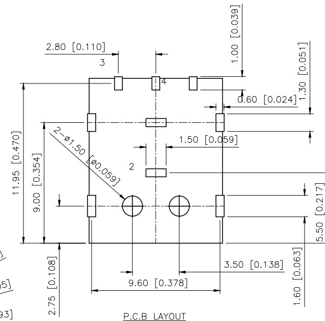
P.C.B LAYOUT
