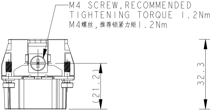
TYPE I, T2040062101-000, WITH LOGO 类型 I, T2040062101-000, 带LOGO
