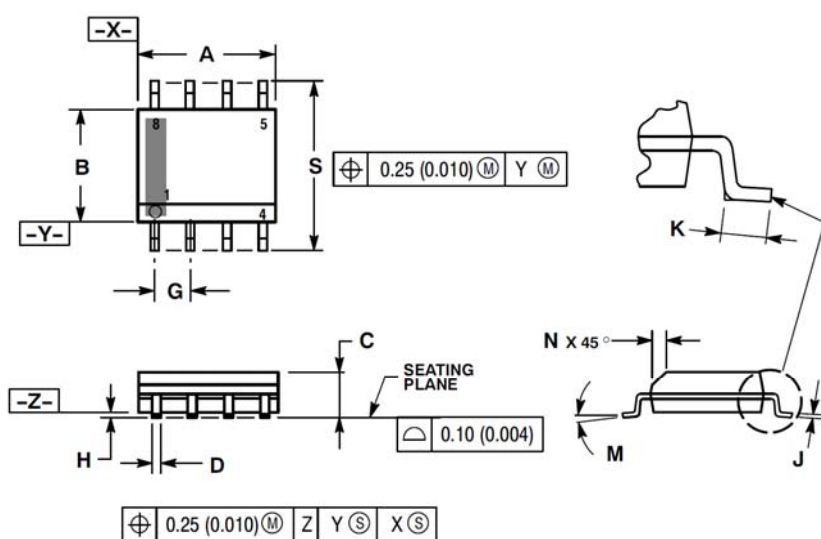
SOP8(SOIC-8)
