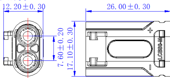
产品尺寸
