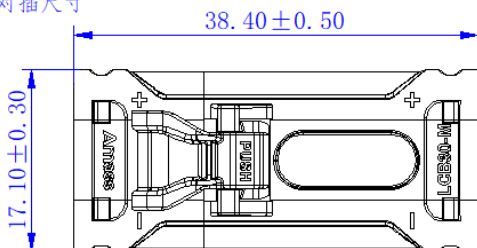
对插尺寸
