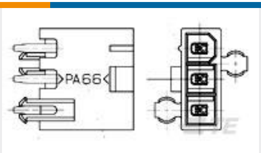
TE Part #2029054-3 3P VAL-U-LOK SR HDR SN V2 W/DH
