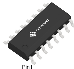
SOP-16
