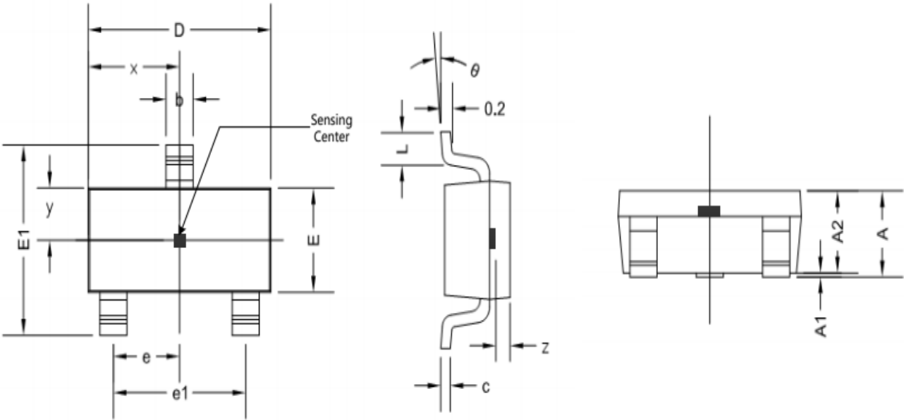
SOT-23封装尺寸
