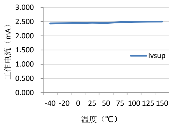
不同温度, 不同工作电压下, 电源电流特性曲线
