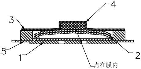
A-A
