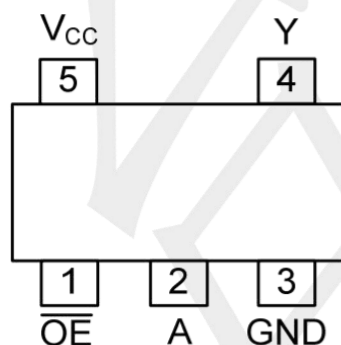
SOT23-5 / SOT353
