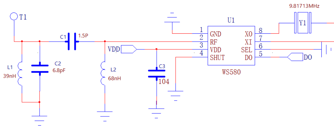
图1 315MHz 1.5kbps典型电路
