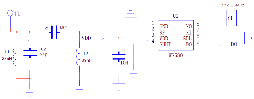
图2 433.92MHz 1.5kbps典型电路
