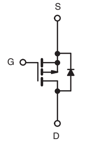
P-Channel MOSFET
