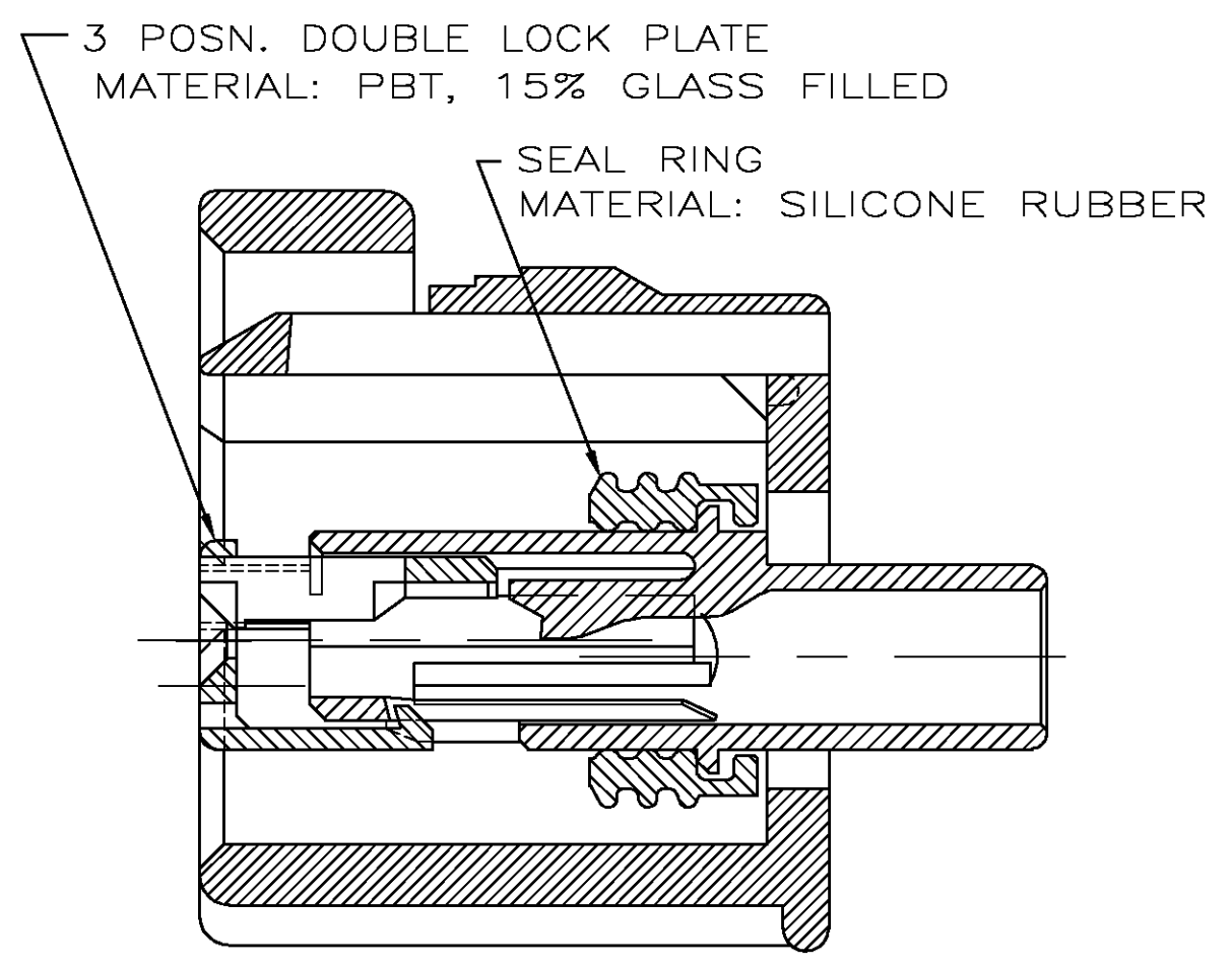
SECTION A-A
