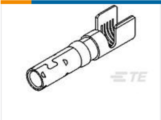
TE Part #213843-4 PWRBAND SKT CNT ASSY,8-10,L.P.
