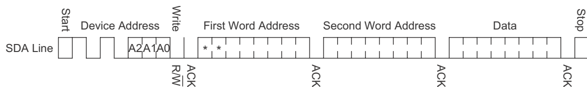
Byte Write Timing
