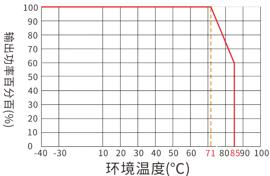
温度降额曲线图
