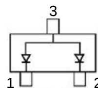
BAT54CW
