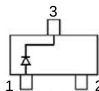
BAT54W
