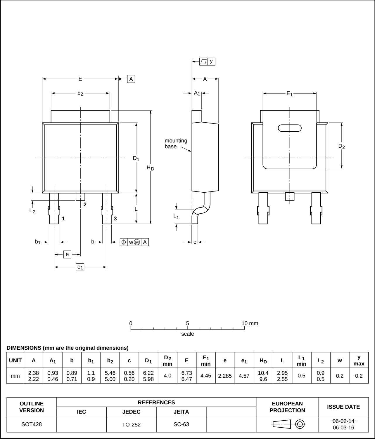
Fig 17. DPAK (SOT428)
