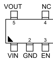
SOT23-5
