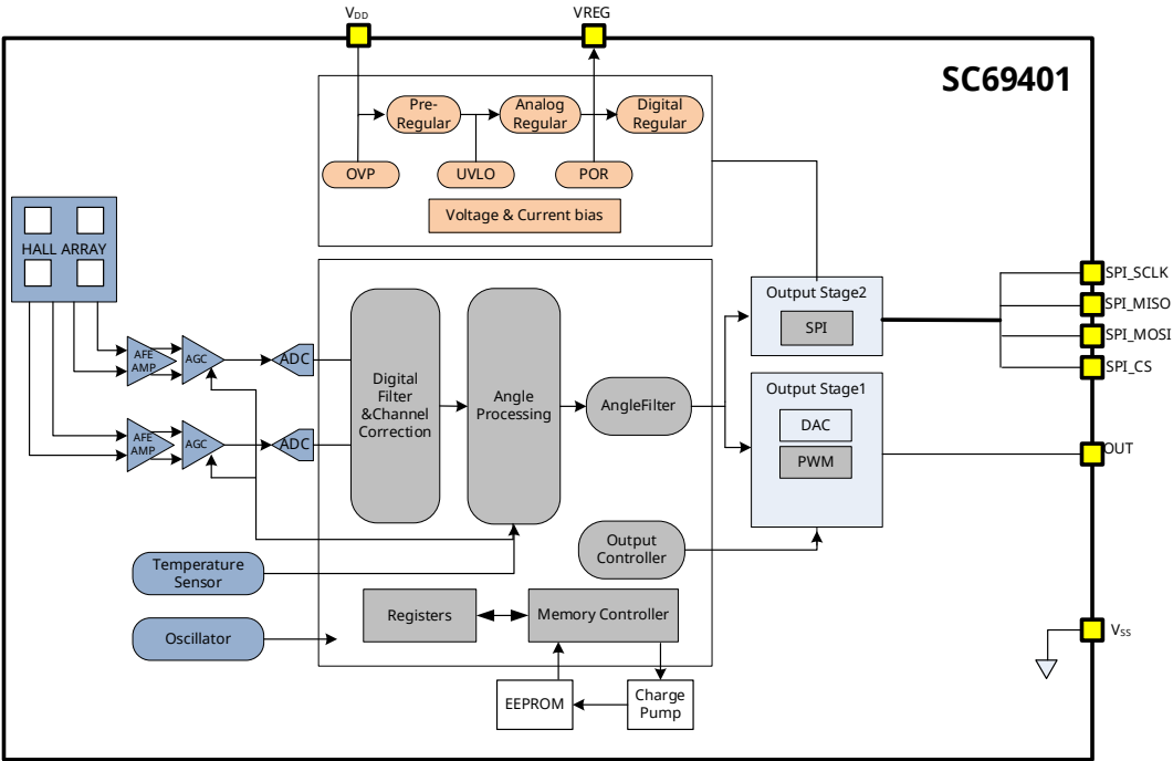
图8 功能框图
