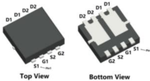
PDFN3X3-8L
