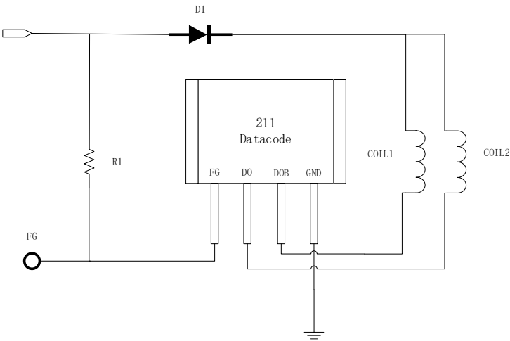
图 4 典型应用电路
