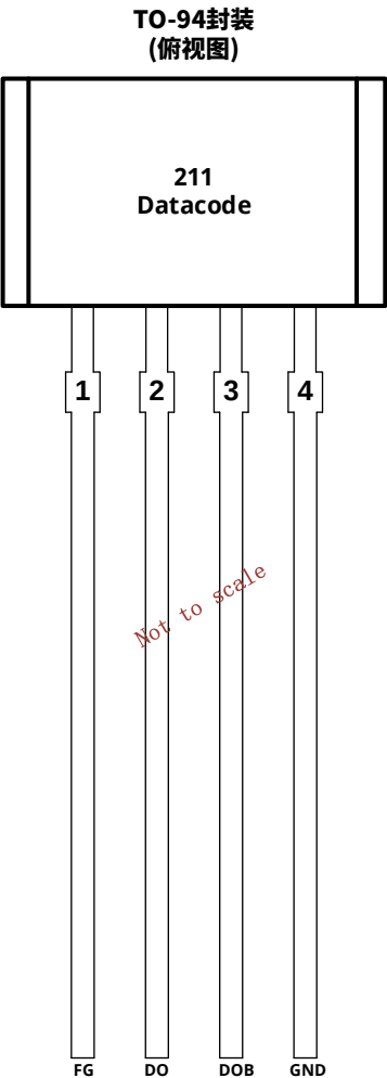
图 2 引脚描述
