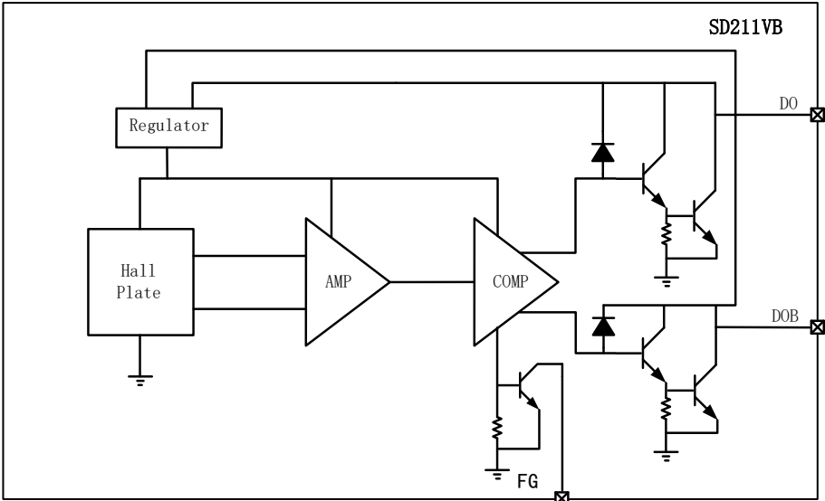
图 3 功能框图
