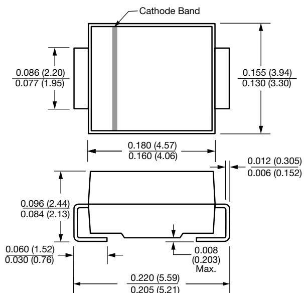
SMB (DO-214AA)
