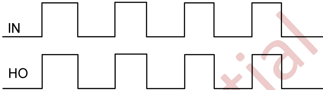
图 9-1 输入输出时序波形
