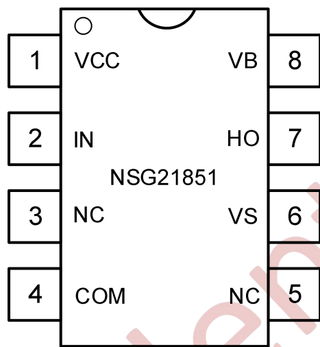
图 7-1 8-脚 SOP 顶视图
