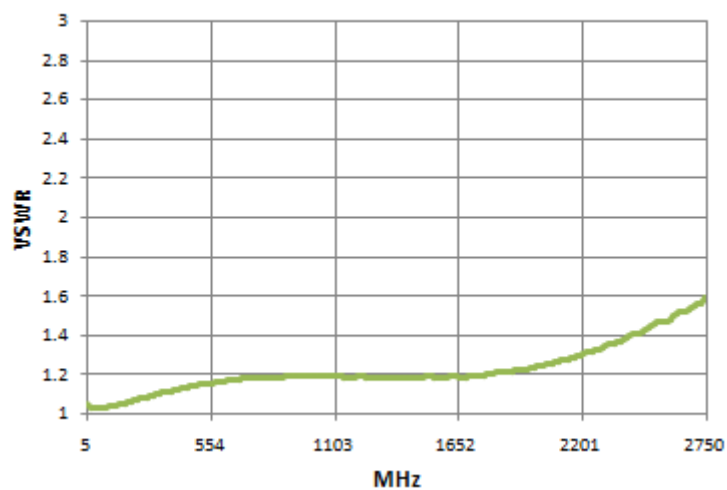
VSWR-S
