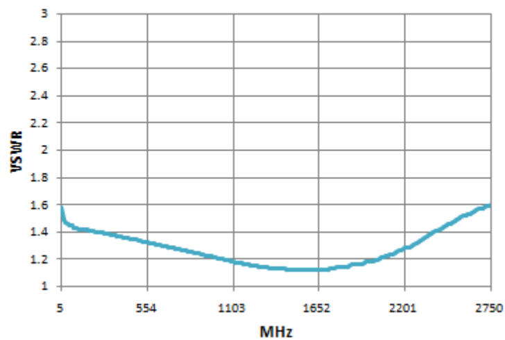
VSWR-2
