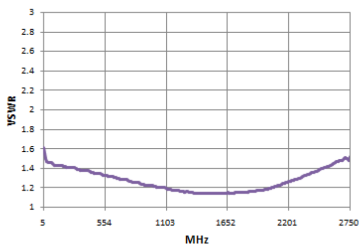
VSWR-1
