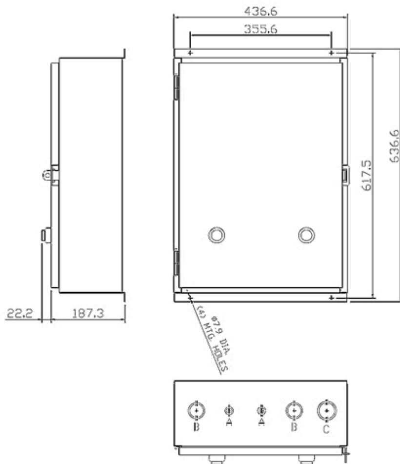
CONDUITS TYP. TOP & BOTTOM
