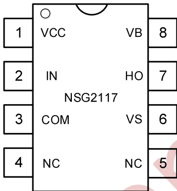
图 7-1 8-脚 SOP8 顶视图
