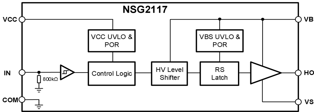
图 10-1 NSG2117 的功能框图
