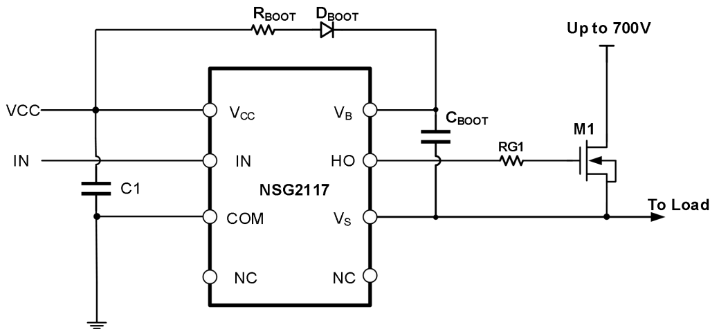
图 10-2 NSG2117 典型应用电路图
