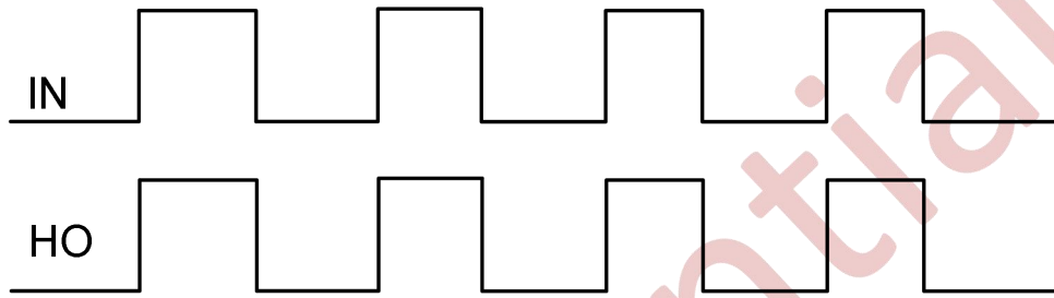
图 9-1 输入输出时序波形
