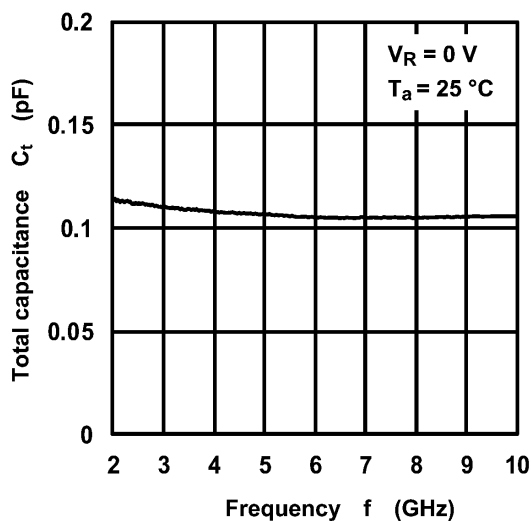
Fig. 7.4 C_t - f
