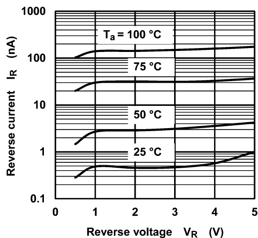
Fig. 7.2 I_R - V_R
