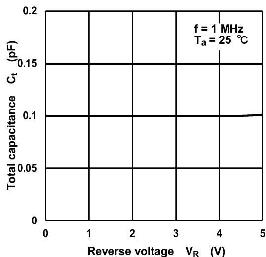
Fig. 7.3 C_t - V_R
