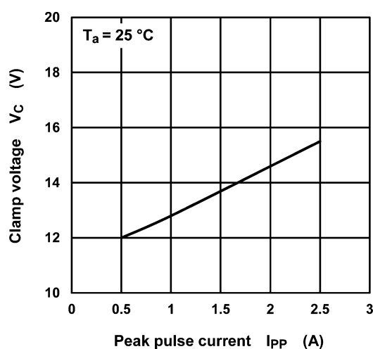
Fig. 8.1 V_C - I_{PP}
