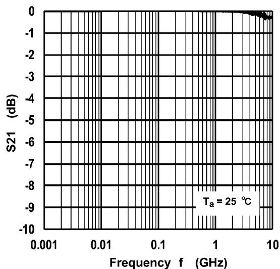
Fig. 9.1 S_{21} - f
