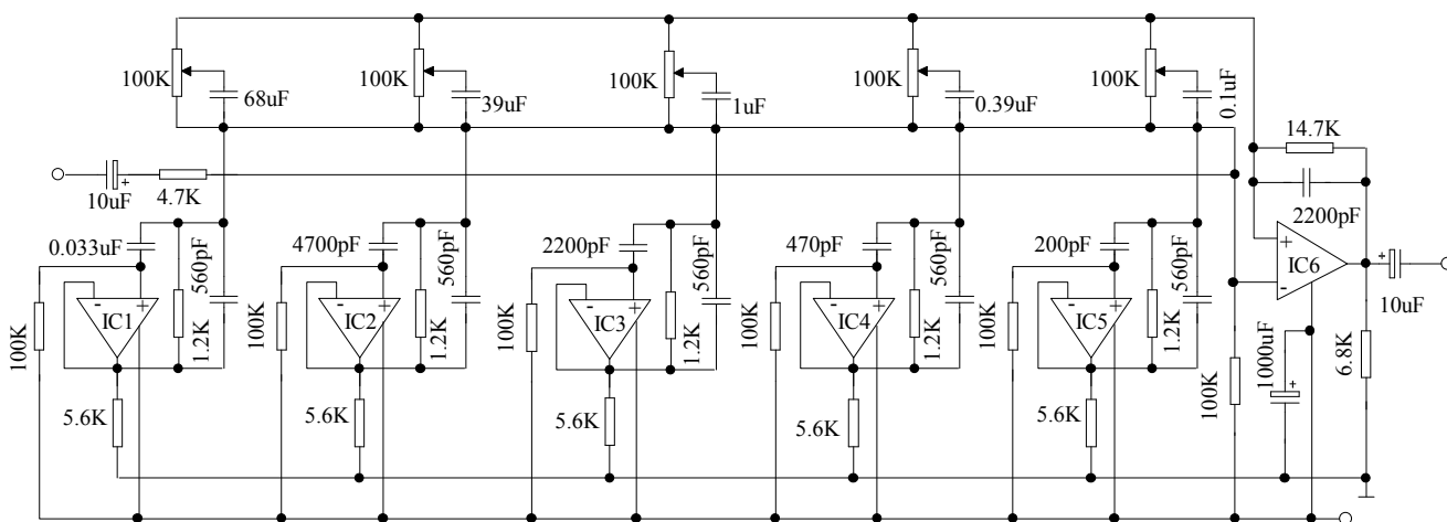
用于五频率音调控制电路
