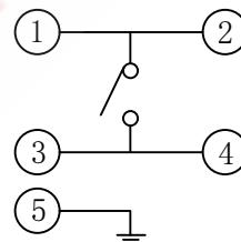
电路图 CIRCUIT DIAGRAM
