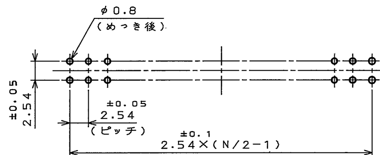
基板取付穴寸法(参考)
