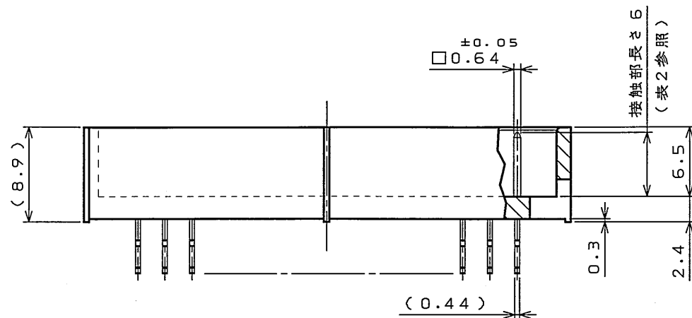
SECT. A-A (SCALE 5:1)
